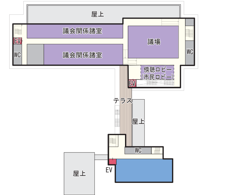
4階平面図
