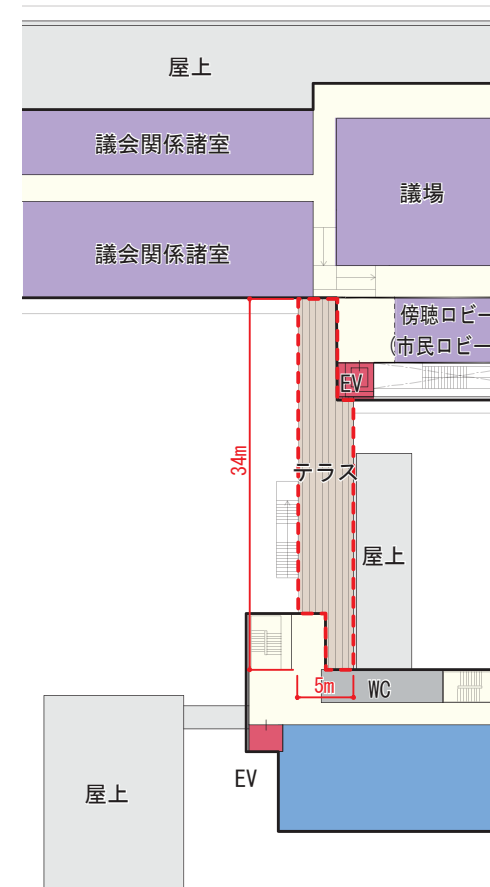
○ 4階平面図
