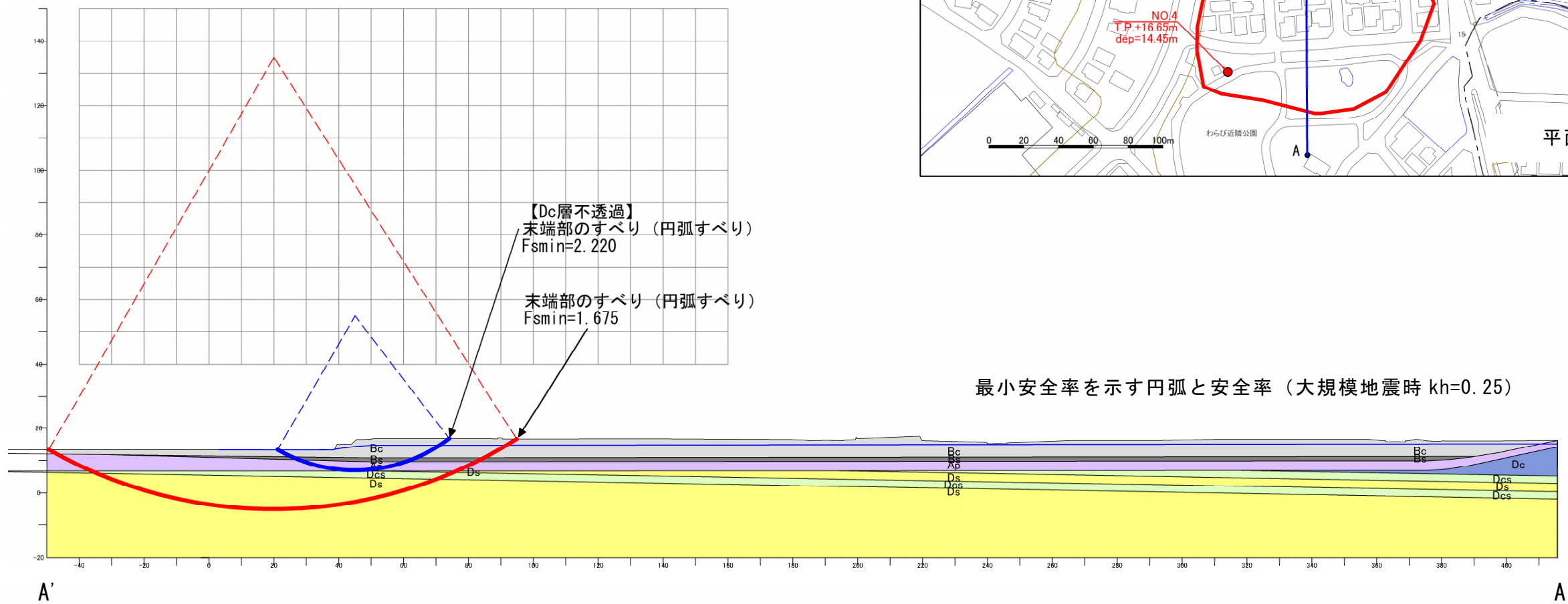
図-7.4.2 四街道市 0064 における安定解析の結果
