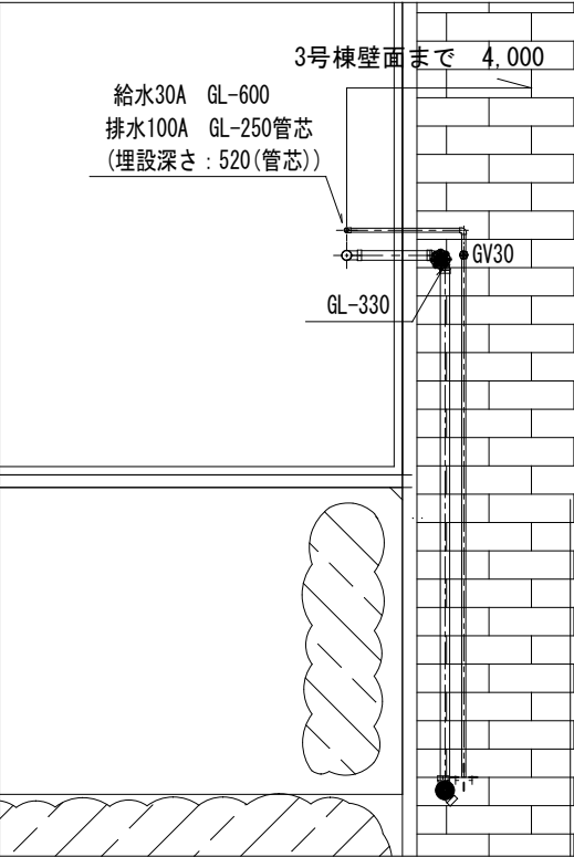
給排水部分拡大 S = 1 : 100
