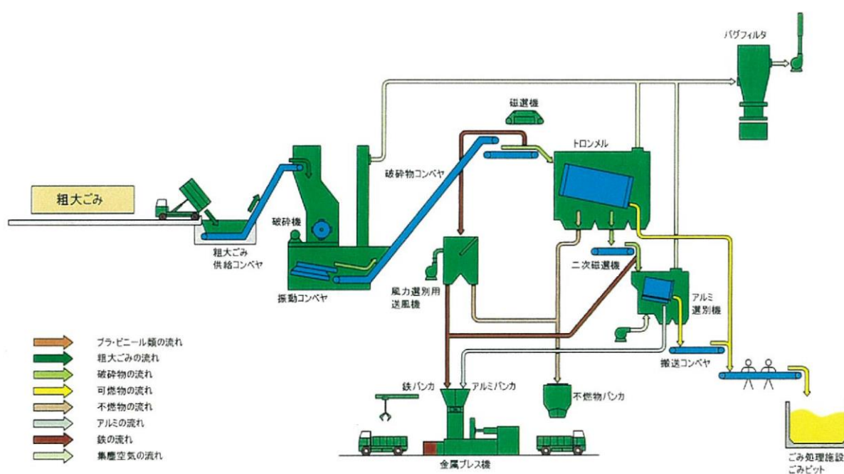
図 2-1 現施設（粗大ごみ処理ライン）の概要
