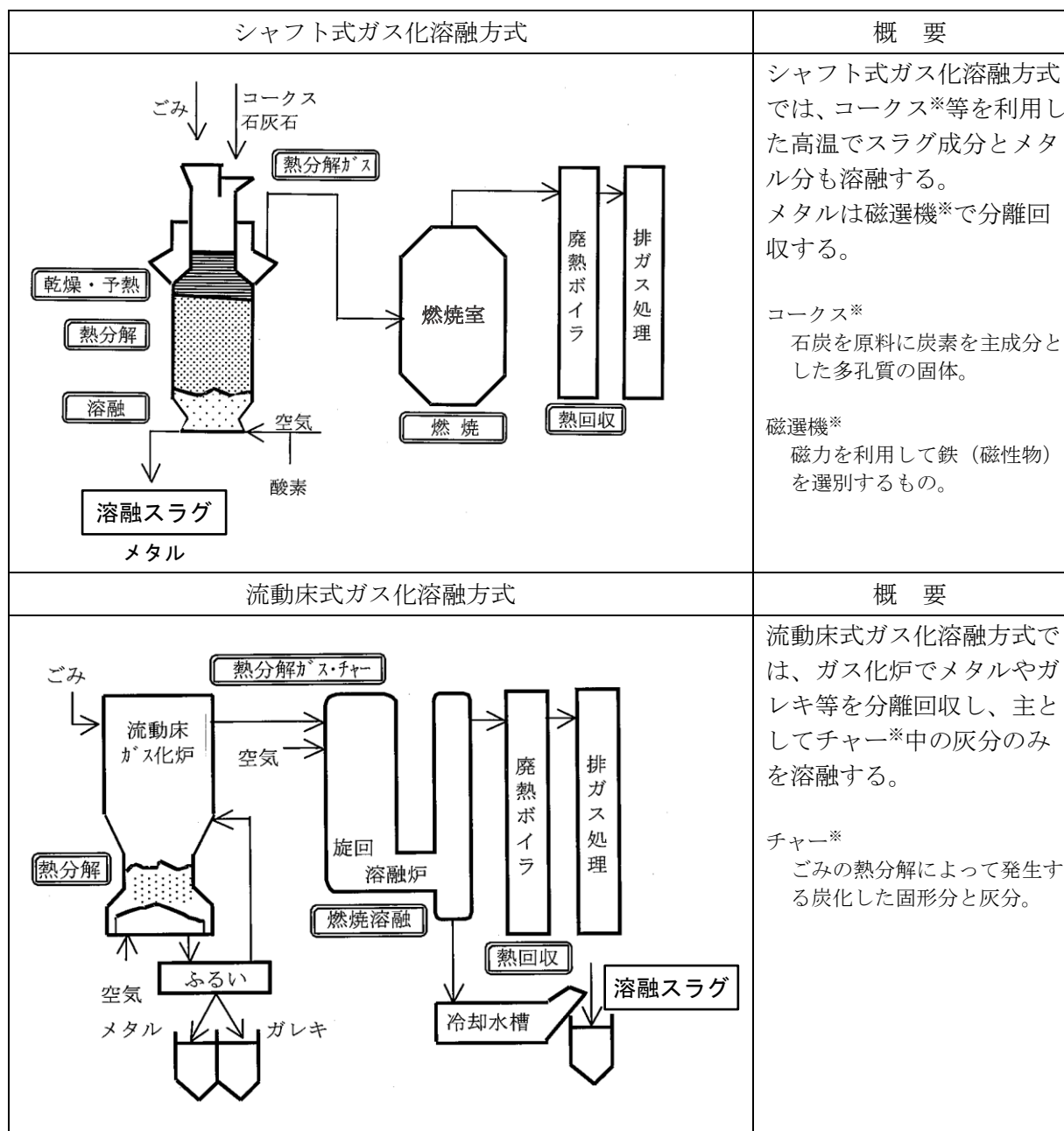
図 1-2 ガス化溶融方式の概要
