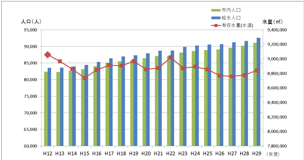
図 3.2 給水人口と需要量の推移
