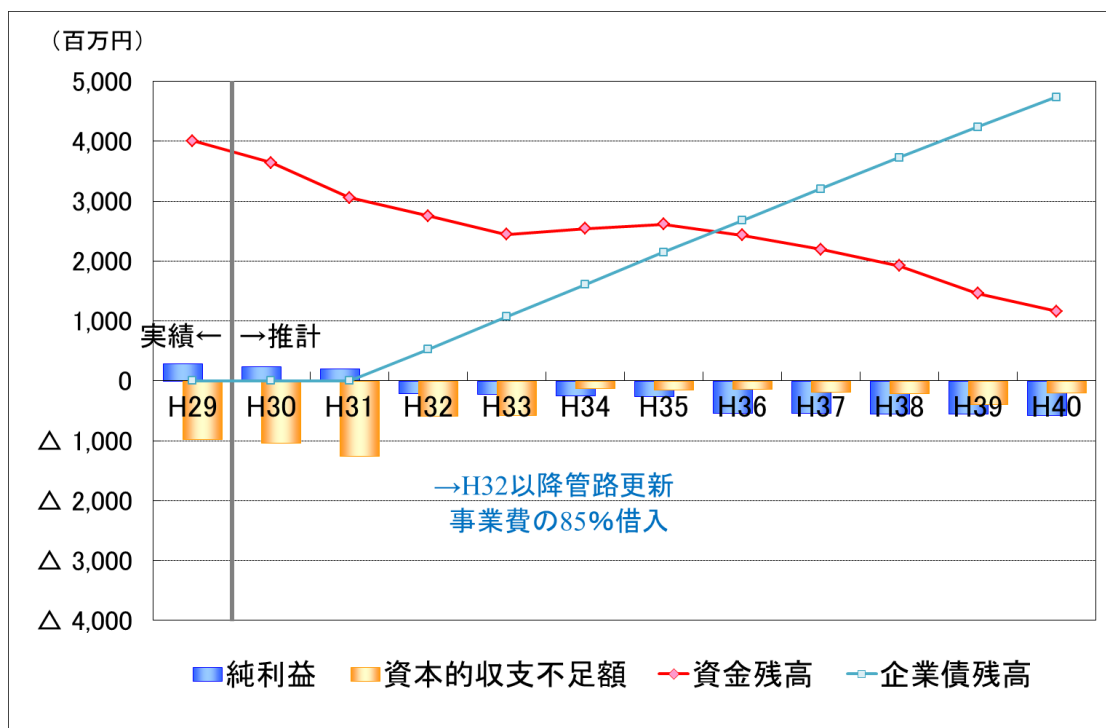
図 3.10 財政状況の見通し（水道事業）（企業債借入あり）
