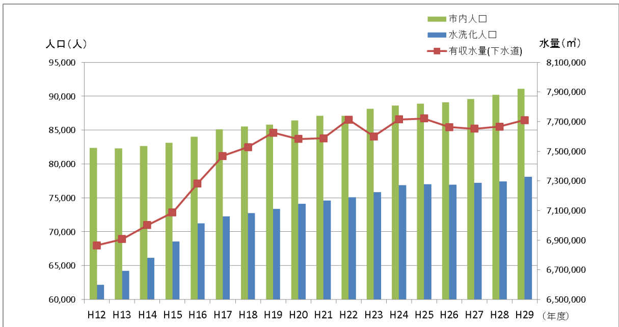
図 3.3 水洗化人口と需要量の推移
